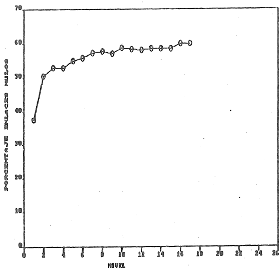
Figura 8 "Distribución de enlaces nulos por niveles en la parte-árbol con n=4"
