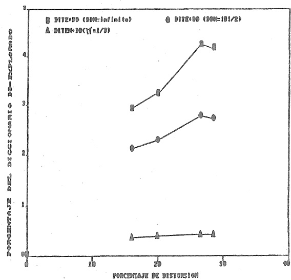
Figura 17 "Gráfica del porcentaje promedio del diccionario implicado en el cálculo de DD en los esquemas DITE+DD y DITEM+DD"
