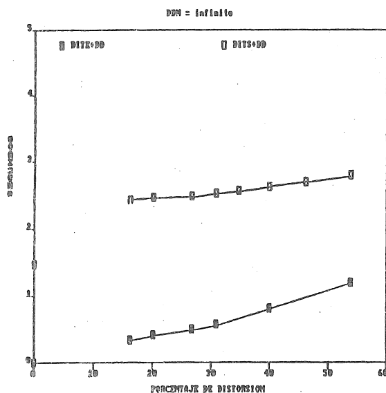
Figura 14 "Gráfica de los tiempos promedio de búsqueda para los esquemas DITS+DD y DITE+DD"
