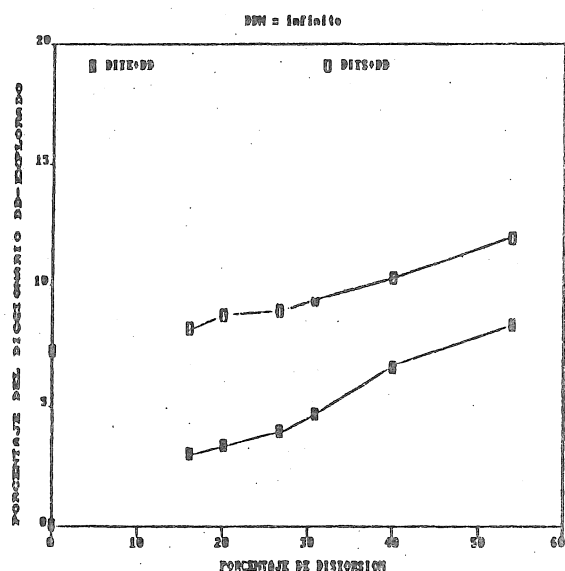
Figura 15 "Gráfica del porcentaje promedio del diccionario implicado en el cálculo de DD en los esquemas DITS+DD y DITE+DD"
