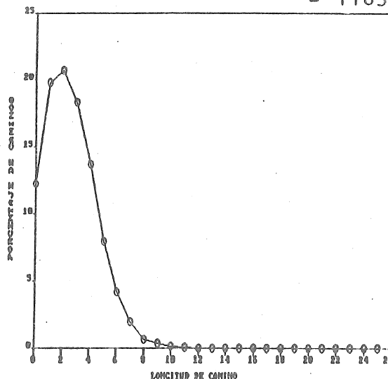
Figura 11 "Gráfica de la distribución de las longitudes de los caminos en la parte-cadena"
